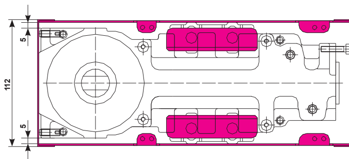
Fissaggio del corpo alla cassetta a cementare Body fixed to the cement case Fijación del cuerpo a la caja a cementar
